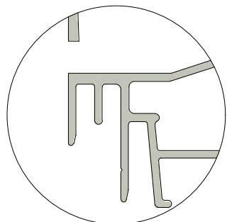
Weep hole ( 1 : 1 )
